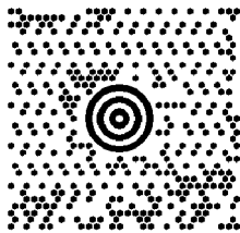
Maxicode
